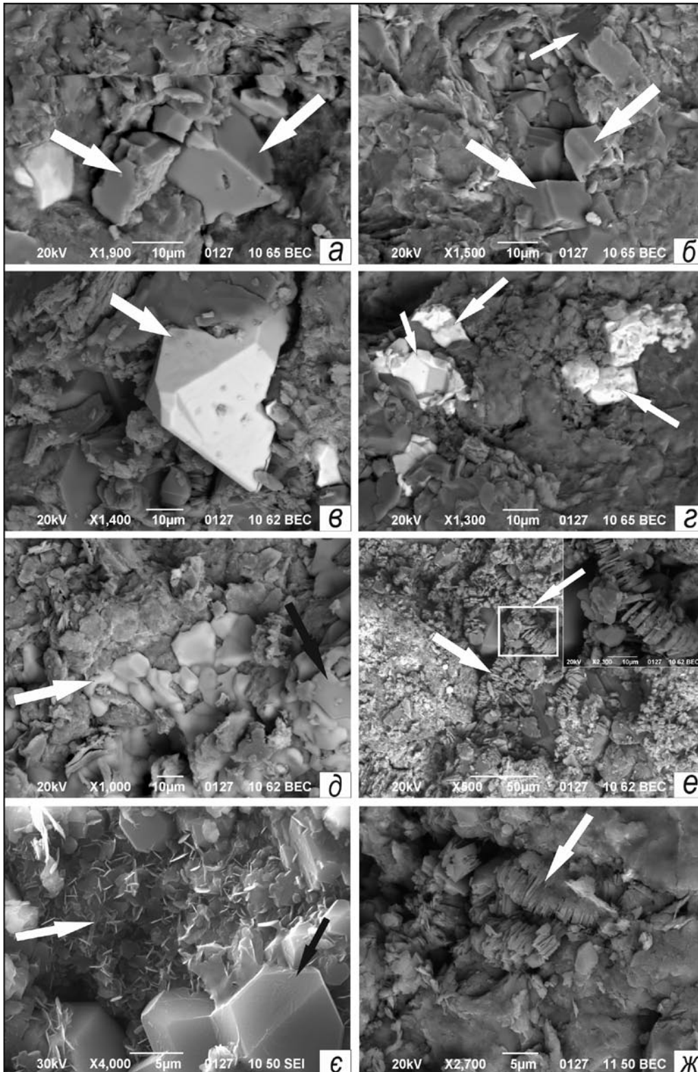
Рис. 6. Електронномікроскопічні знімки мінеральних новоутворень а — ангідрит, св. Кобзівська-50 (12/1) (гл. 3369–3373 м, алевроаргіліт червоноколірний); б — доломіт, св. Кобзівська-50 (12/1) (гл. 3369–3373 м, алевроаргіліт червоноколірний); в — барит, Кобзівська-50 (15/1) (гл. 3434–3442 м, пісковик червоноколірний, дрібнозернистий); г — целестин, св. Кобзівська-50 (12/1); д — галіт (біла стрілка), сильвін (чорна стрілка) св. Кобзівська-50 (15/3) (гл. 3434–3442 м, пісковик дрібнозернистий червоноколірний); е — новоутворені текстуровані полікристали каолініту в міжзерновому просторі, Кобзівська-50 (15/1); є — хлорит залістий (біла стрілка), утворення ідіоморфного кварцу (чорна стрілка), св. Кобзівська-50 (15/1); ж — гідрослюдястий агрегат, св. Кобзівська-50 (14/1) (гл. 3412–3416 м, пісковик дрібнозернистий червоноколірний)
