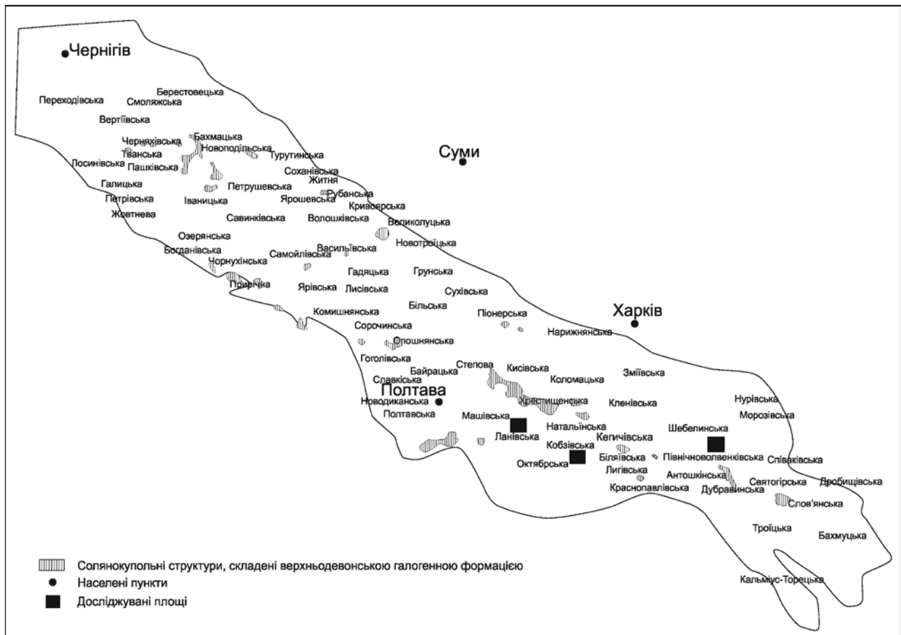
Рис. 1. Схема розташування досліджуваних площ Кобзівської, Ланівської та Північноволвенківської (карта розповсюдження нижньопермської галогенної та теригенної червоноколірної формації ДДЗ [4])
