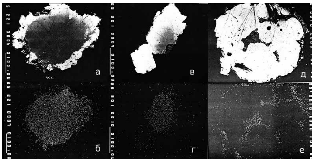
Рис. 2. Рентгеновские снимки зонального золота из донных осадков шельфа Черного моря (район Тендровской косы и Затоки), масштабная метка соответствует 0,1 мм а, в, д — снимки во вторичных электронах; б, г, е — те же образцы в характеристических излучениях по линии L\alpha Ag (б, г) и по линии L\alpha Pb (е).
