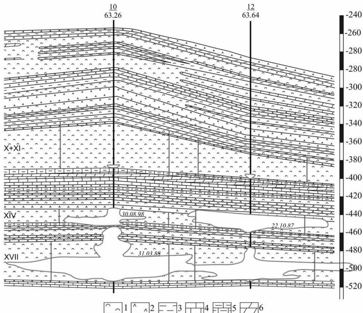
Рис. 2. Розріз через св. 10 та 12 Райгородської ділянки Слов'янського розсолотросту. Спостворена форма камер та їх гідравлічний зв'язок (за матеріалами І. Н. Шевченко, 1952; С. В. Софронів та ін.)
