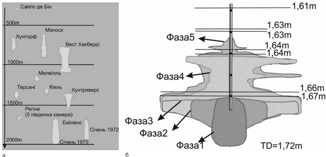
Рис. 1. Приклади форм камер, створених методом вилуговування у різних типах соленосних формацій (перерізи). Зіставлено об'єми ємності Еміненс, яка зазнала конвергенції (а). Зміна форми під час розмиву ємності Регіна (камера 5), що створена у девонській соленосній формації пластової форми залягання (Вінніпег, Канада) (б) [14, 15]
