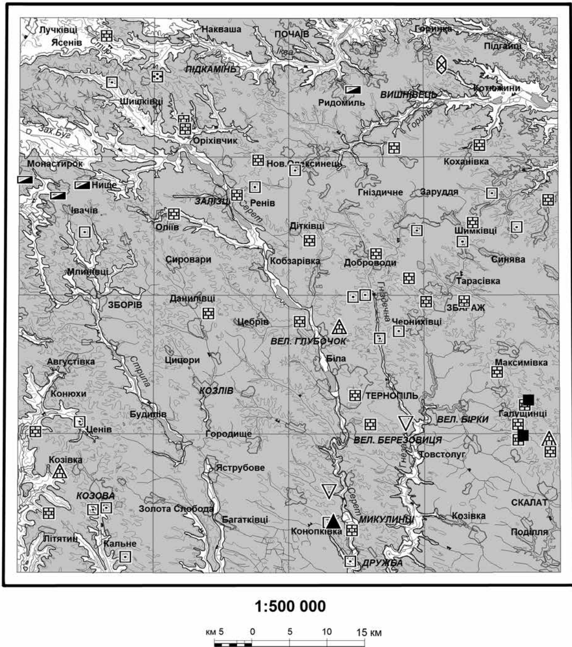
Рис. 2. Корисні копалини міоценових відкладів території досліджень. Масштаб 1 : 500 000. Умовні позначення корисних копалин див. на рис. 1
